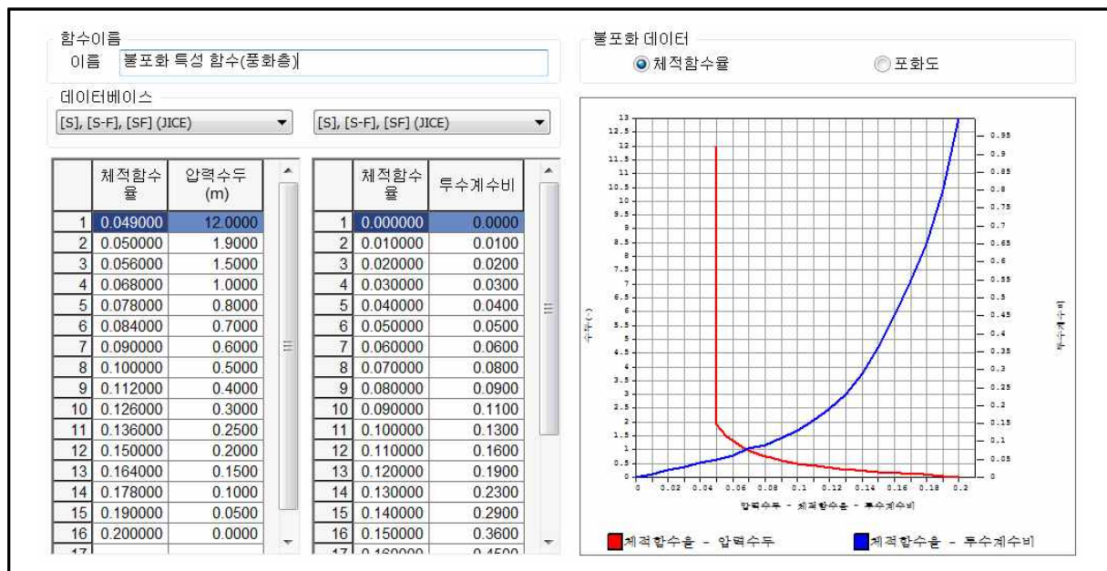
【그림 53-15】 압력수두-채적함수물(포화도)-투수계수비 함수
