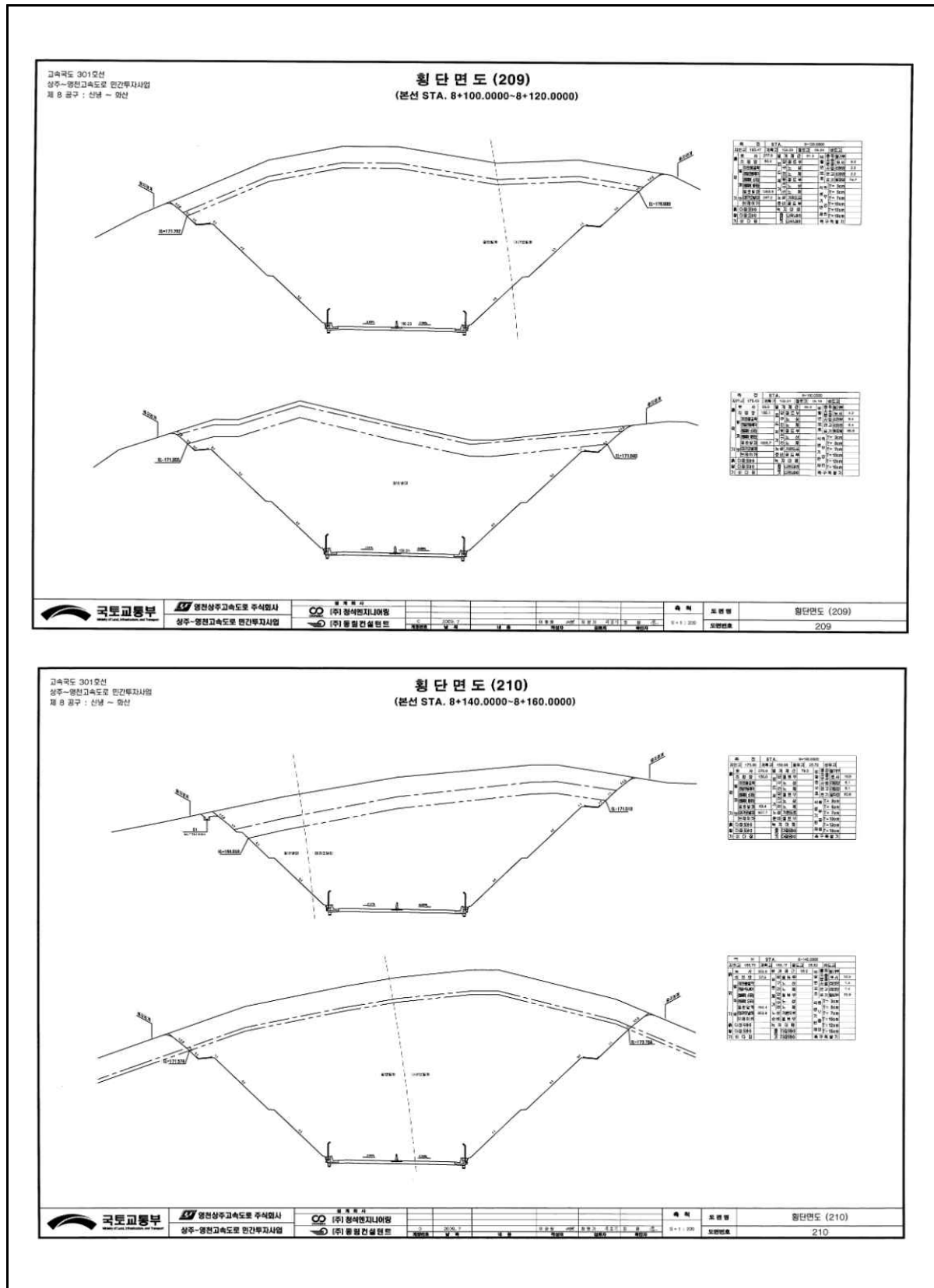
【그림 53-4】 표준횡단면도
